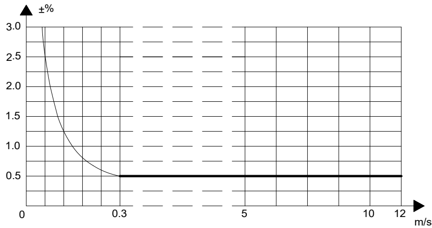
电磁流量计系统的准确性曲线图
