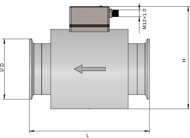
卡箍连接
