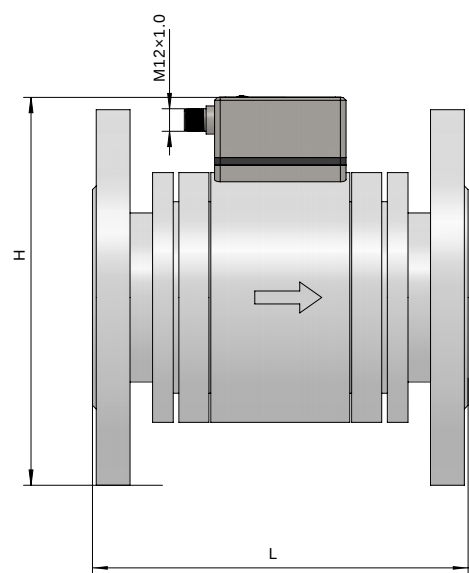
法兰连接
