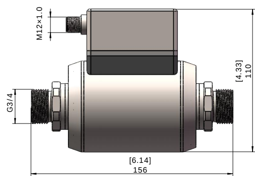
外螺纹连接
